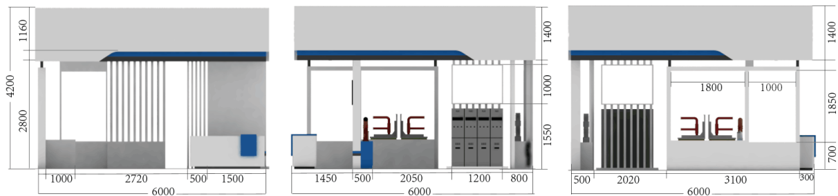
●立面图(单位mm)
